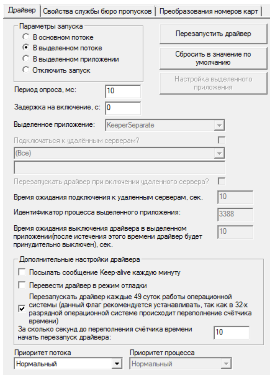
Рисунок 12 — Частные свойства элемента Служба бюро пропусков
