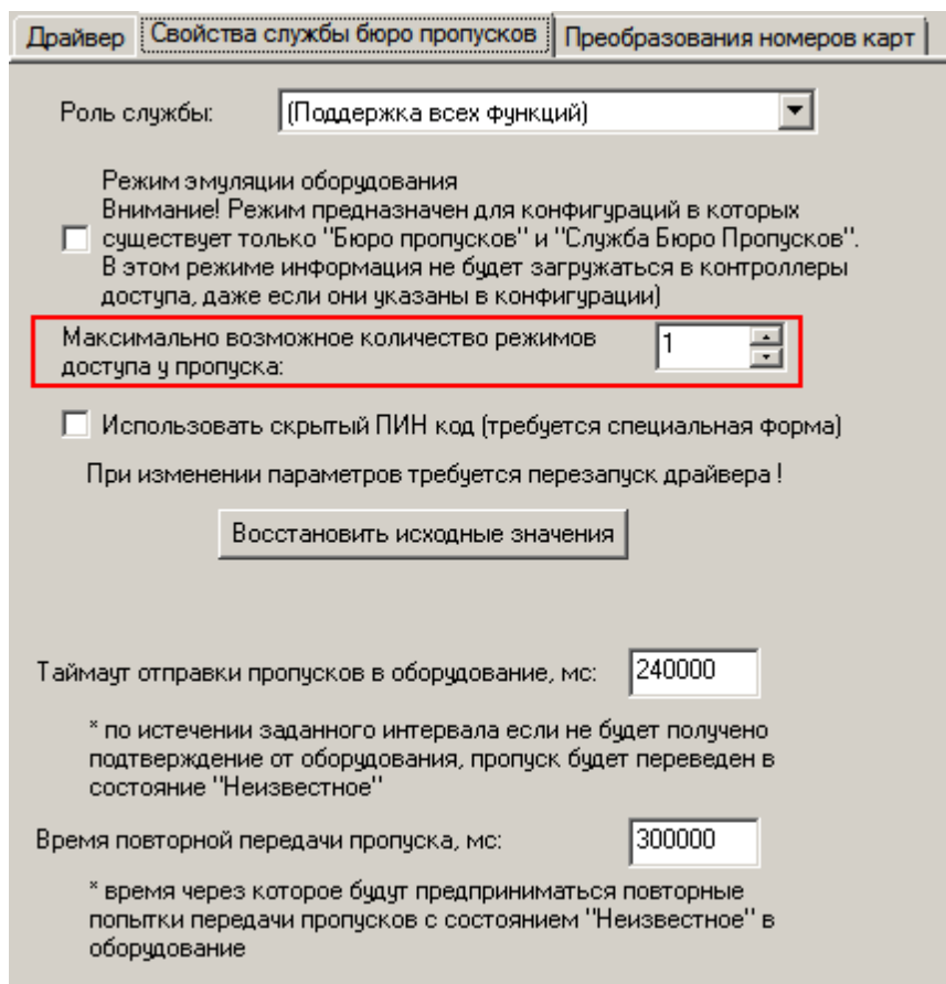
Рисунок 98 – Вкладка Свойства службы бюро пропусков
