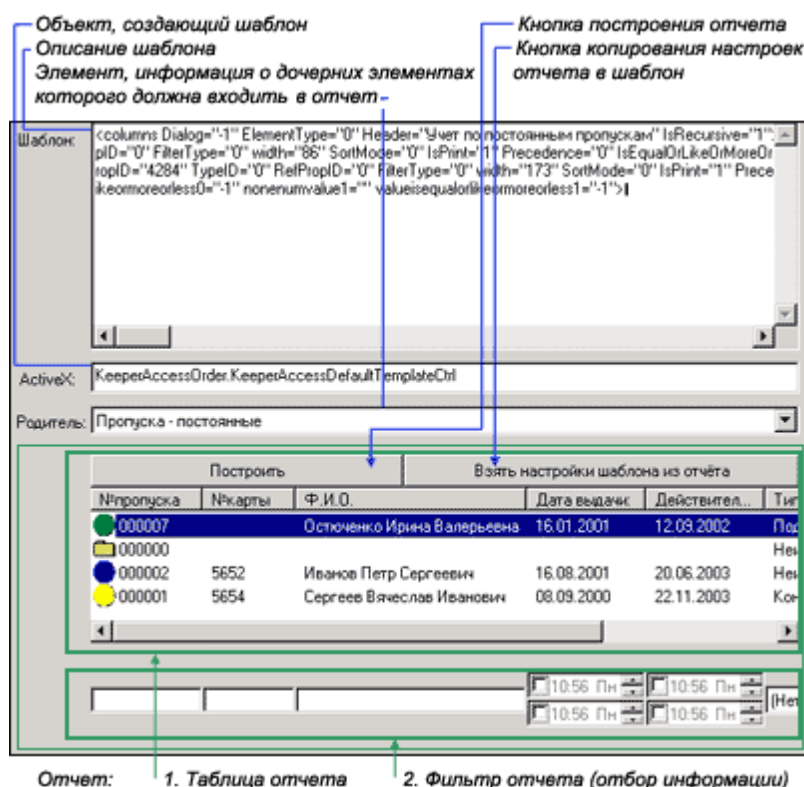
Рисунок 83 — Вкладка Шаблон для отчета
