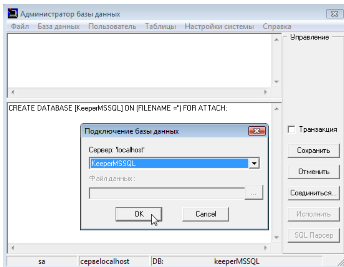
Рисунок 27 — Программа «Администратор MSQL», окно Подключение базы данных
