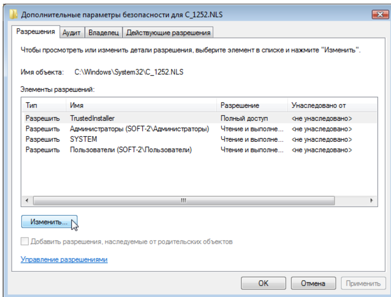
Рисунок 38 — Окно Дополнительные параметры безопасности для C_1252.NLS , вкладка Разрешения
