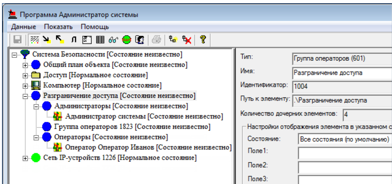
Рисунок 109 — Добавление группы операторов
