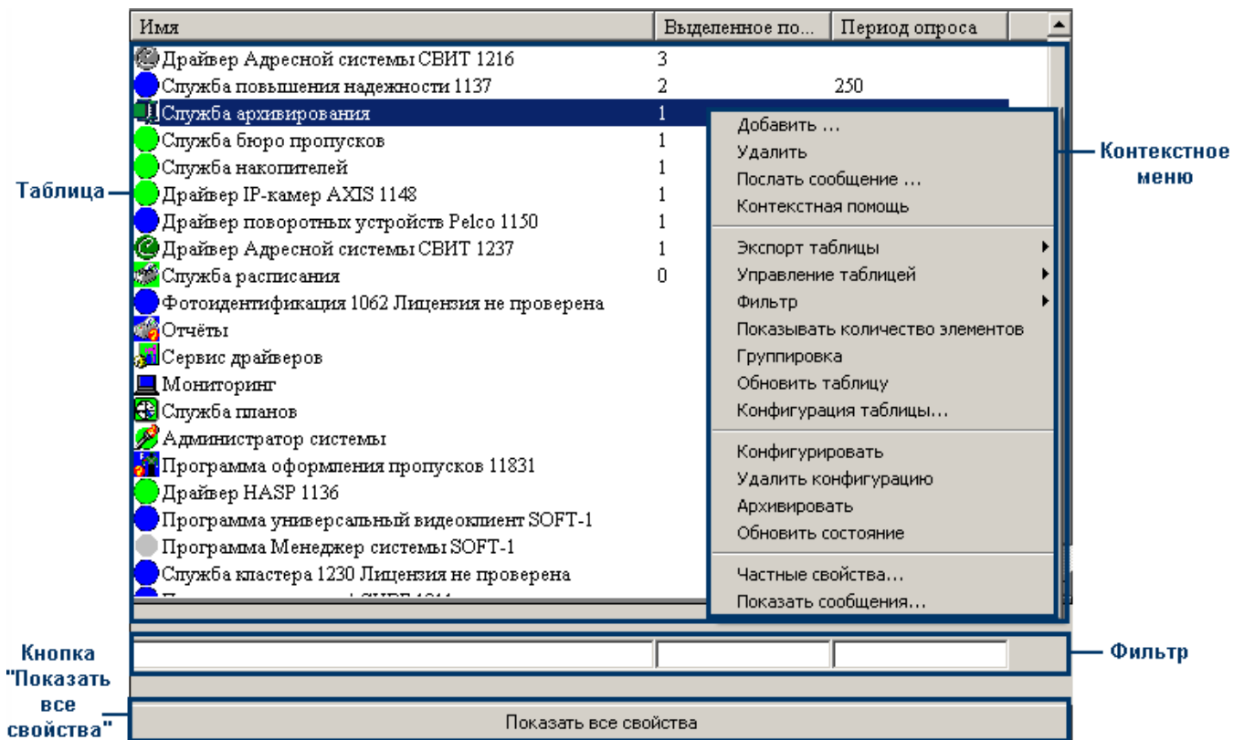
Рисунок 136 — Окно свойств в режиме отображения свойств элемента
