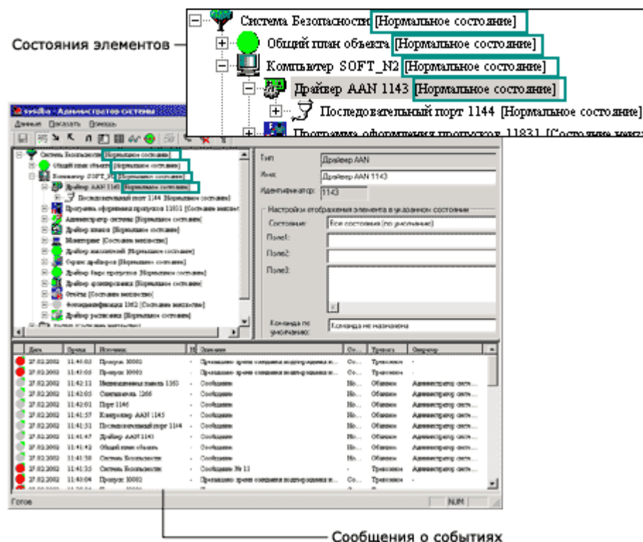
Рисунок 3 — Пример состояний и сообщений
