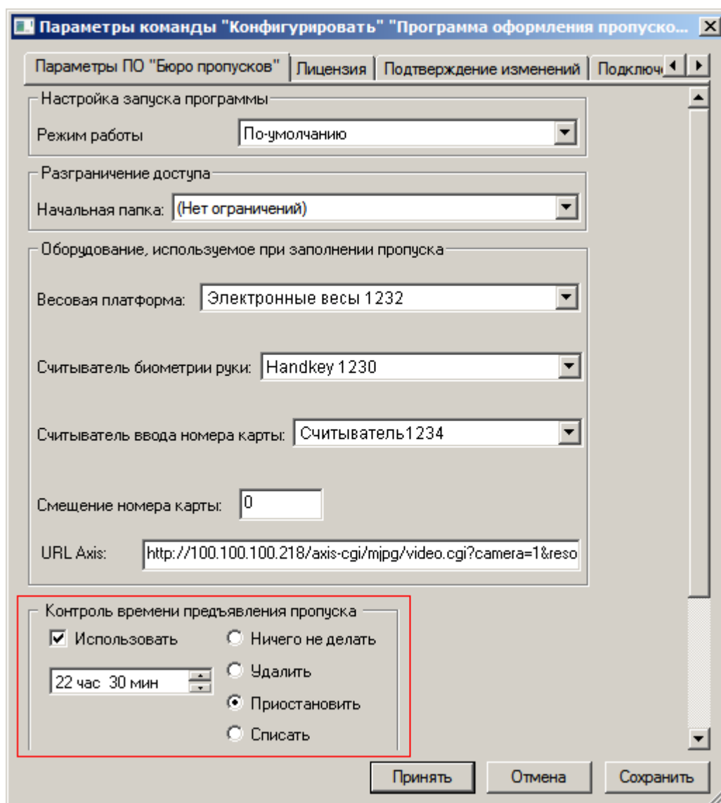
Рисунок 101 — Настройка контроля времени предъявления пропуска
