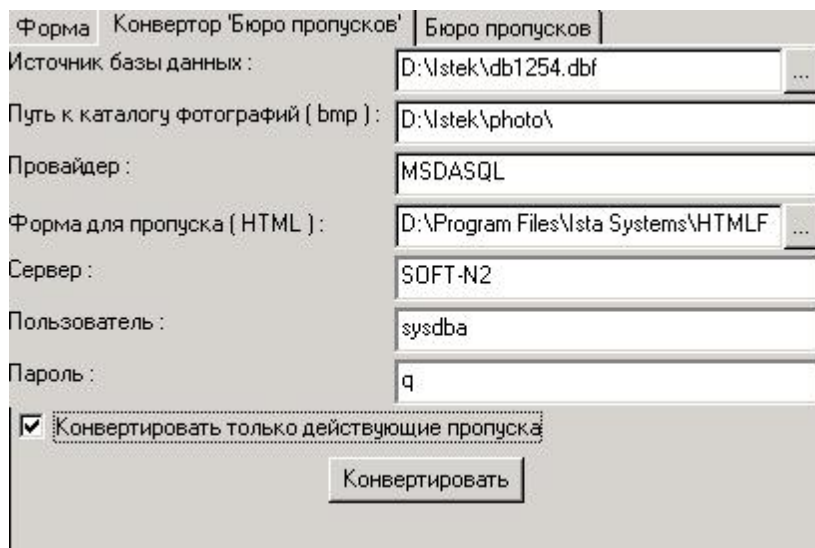
Рисунок 99 — Вкладка Конвертор Бюро пропусков
