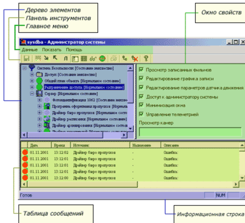
Рисунок 125 — Основное окно программы
