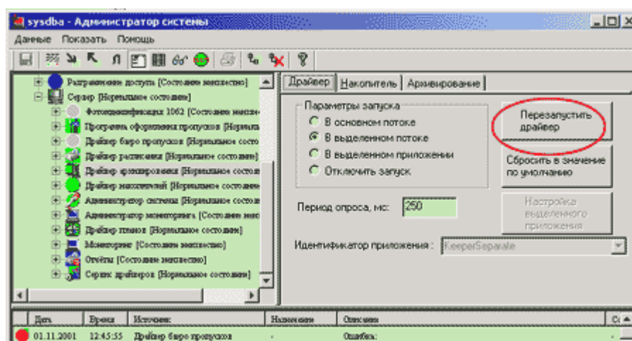
Рисунок 146 — Перегрузка конкретного драйвера
