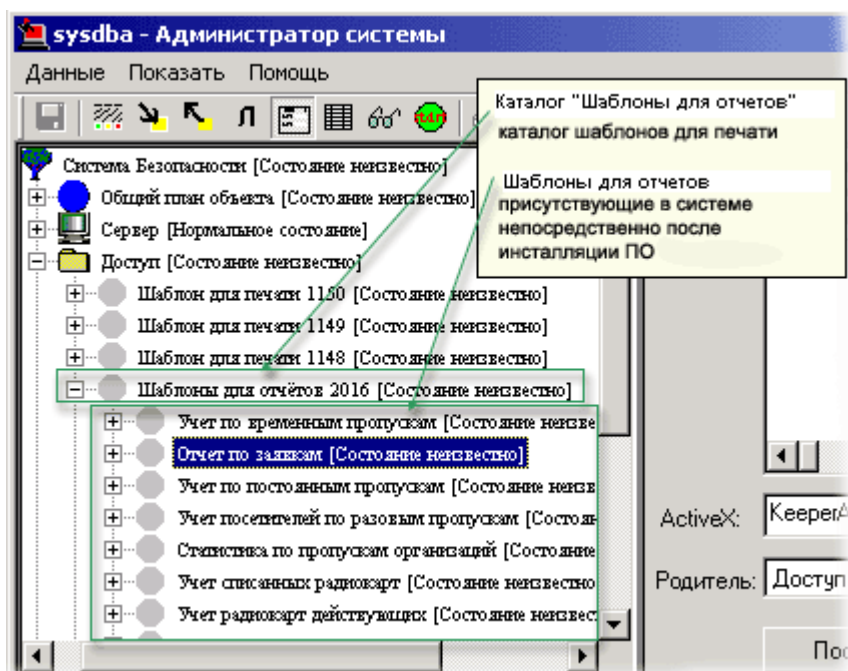
Рисунок 95 — Элементы, представляющие шаблоны для отчетов
