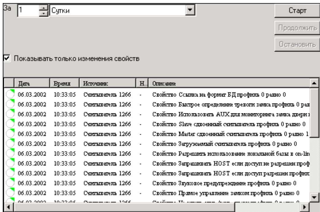
Рисунок 138 — Окно свойств в режиме отображения свойств элемента
