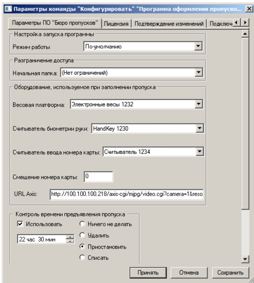
Рисунок 19 — Выбор устройств считывания веса и биометрии
