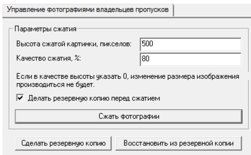
Рисунок 38 — Частные свойства элемента Доступ вкладка Управление фотографиями владельцев пропусков
