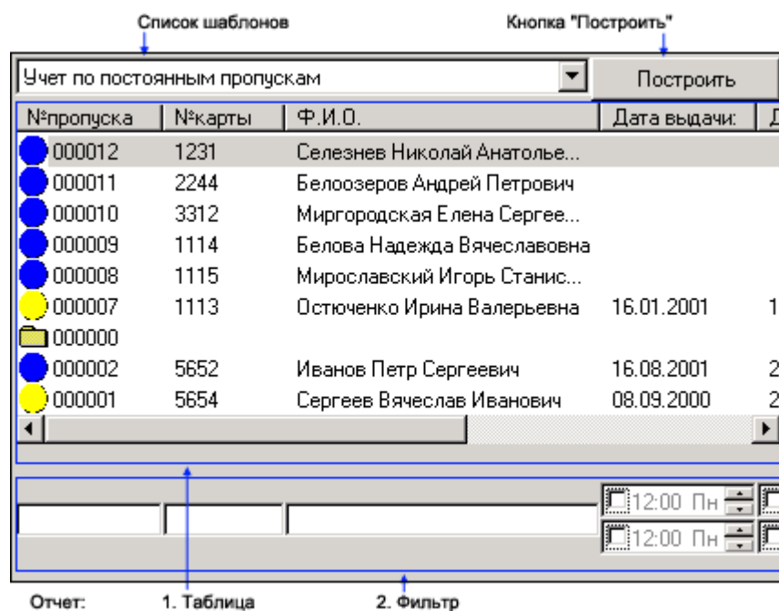
Рисунок 97 — Вкладка Отчеты подсистемы доступа
