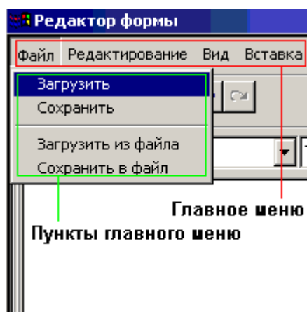
Рисунок 77 — Главное меню «Программы оформления пропусков»
