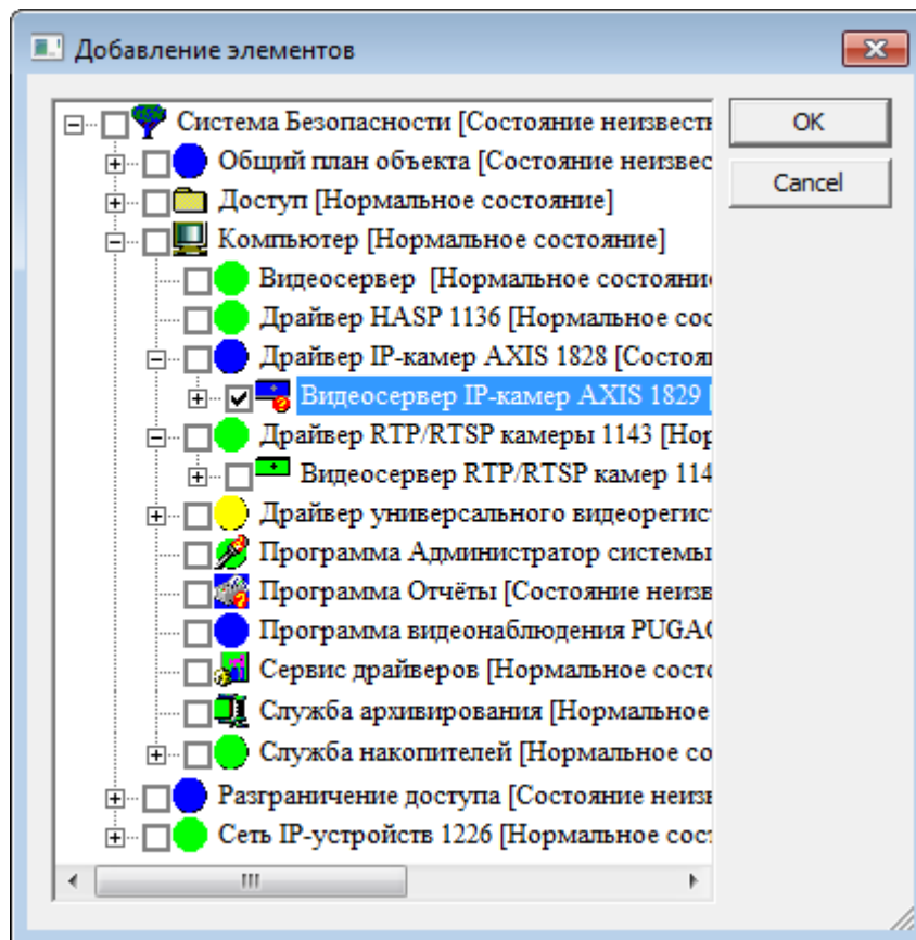
Рисунок 115 — Добавление источников тревог
