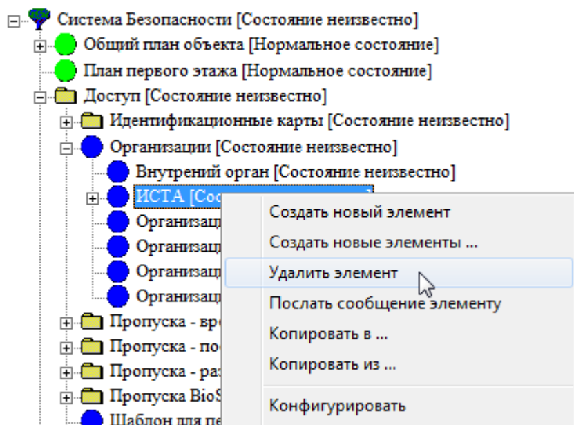
Рисунок 42 — Элементы, соответствующие организациям. Каталог организаций
