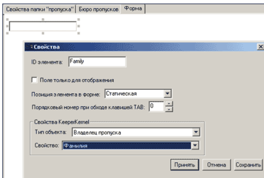
Рисунок 49 — Настройка свойств поля ввода
