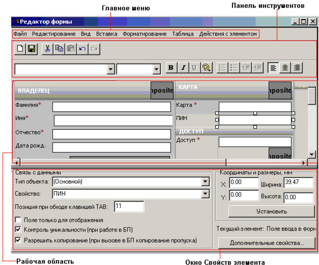
Рисунок 76 — Основное окно Редактора
