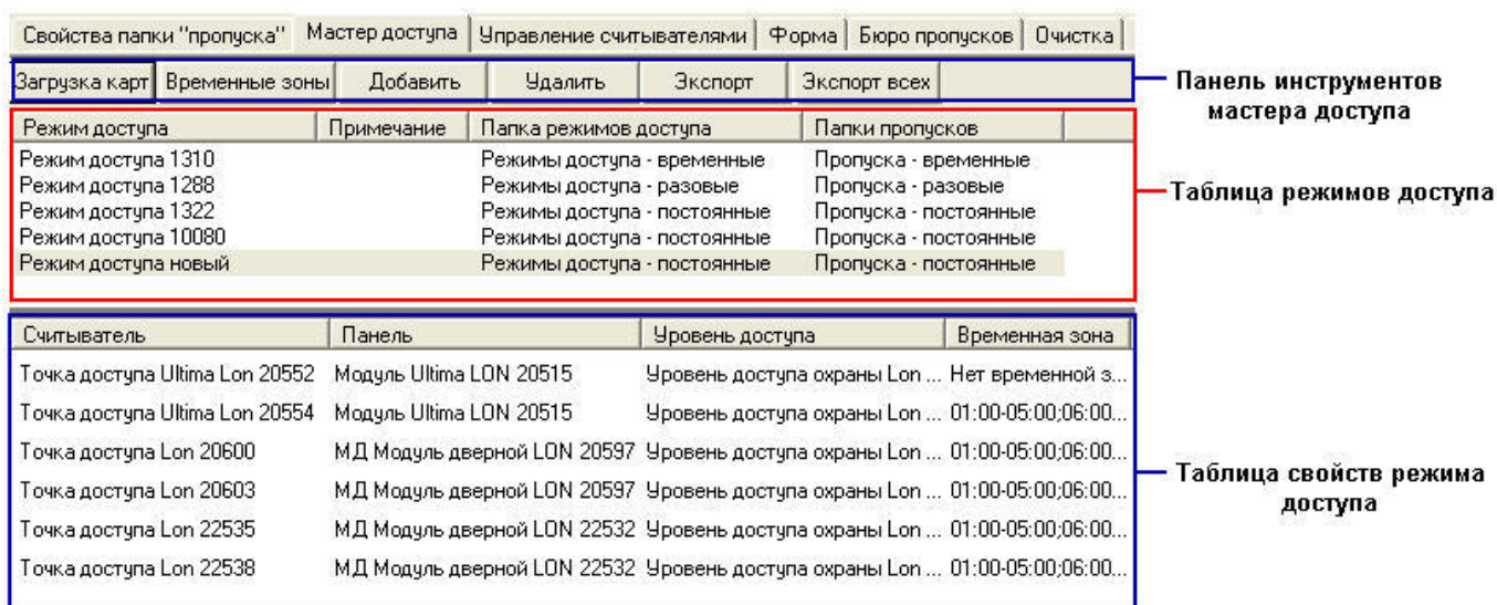
Рисунок 23 — Вкладка Мастер доступа
