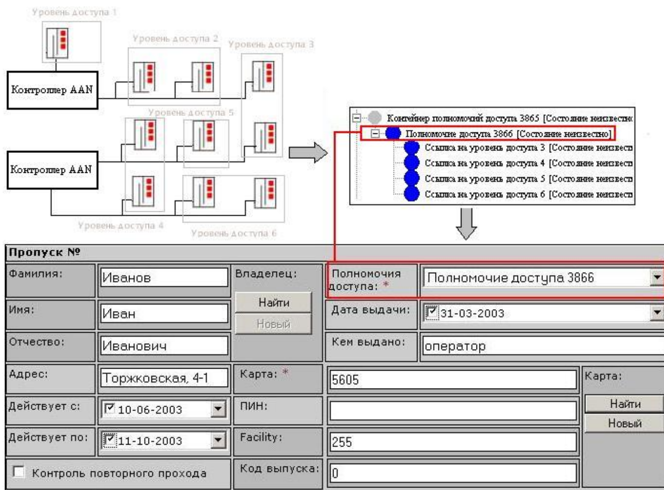
Рисунок 27 — Задание уровней доступа для пропуска
