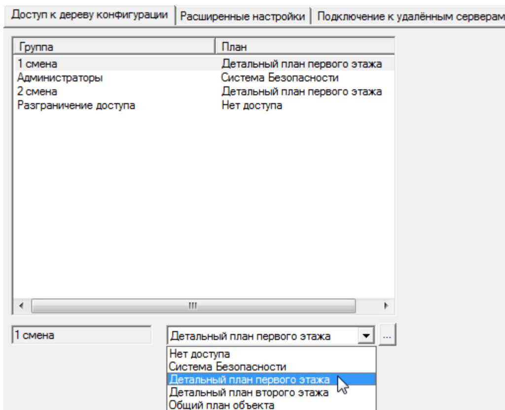
Рисунок 119 — Частные свойства элемента Программа Мониторинг , вкладке Доступ к дереву конфигурации
