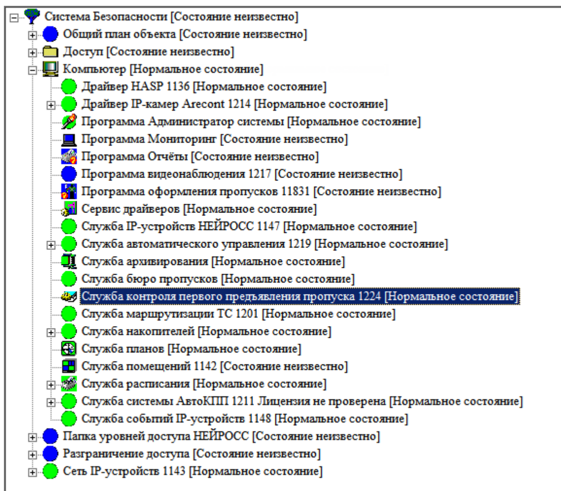
Рисунок 100 — Добавление Службы контроля первого предъявления пропуска
