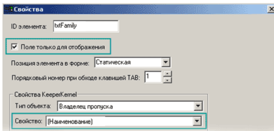
Рисунок 51 — Настройка свойств текста (подписи)
