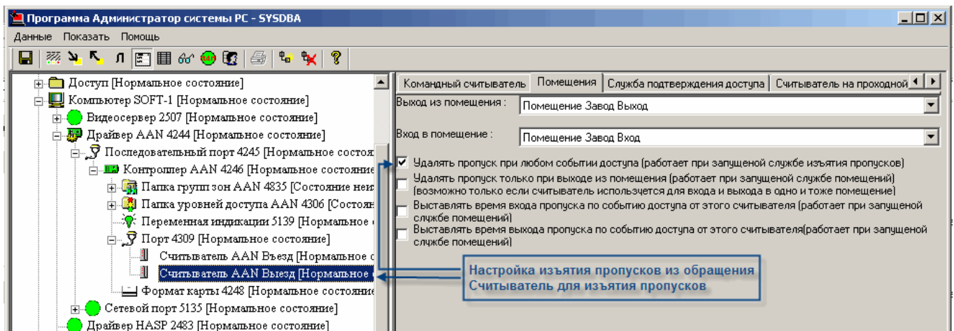
Рисунок 106 — Частные свойства элемента Считыватель , вкладка Помещения
