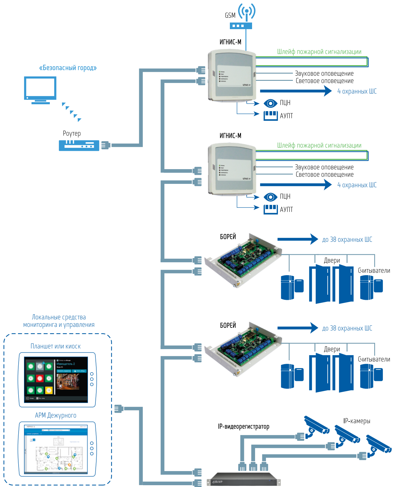
Структурная схема IP-интегрированной комплексной системы безопасности
