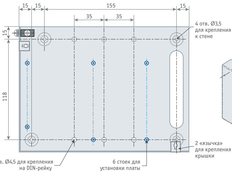
Основание
