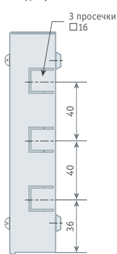
Вид справа
