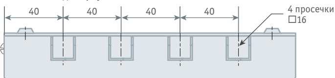
Вид снизу
