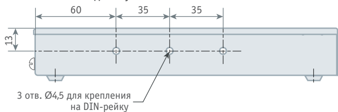
Основание
