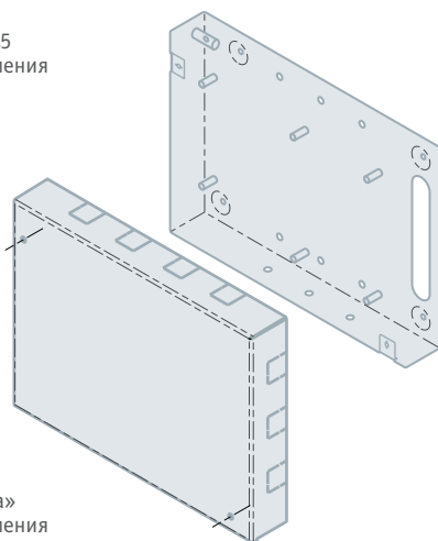
Общий вид
